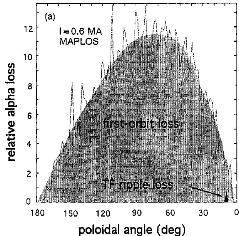
Zweben, NF Fig. 22, TFTR
