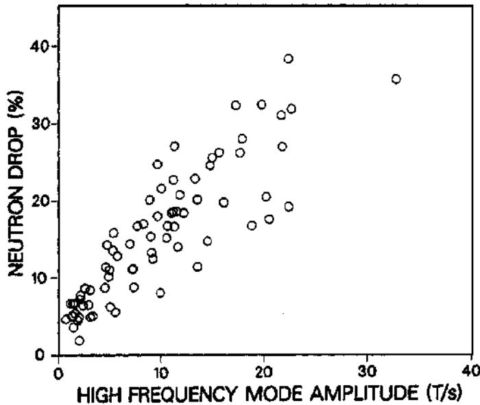
DIII-D (Duong NF 1993 Fig. 8)
